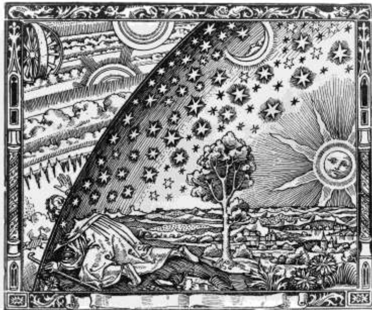
Camille Flammarion: L'Atmosphère. Météorologie Populaire, Paris 1888, S. 163
